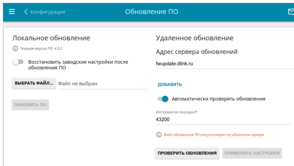
Рисунок 179. Страница Система / Обновление ПО .
