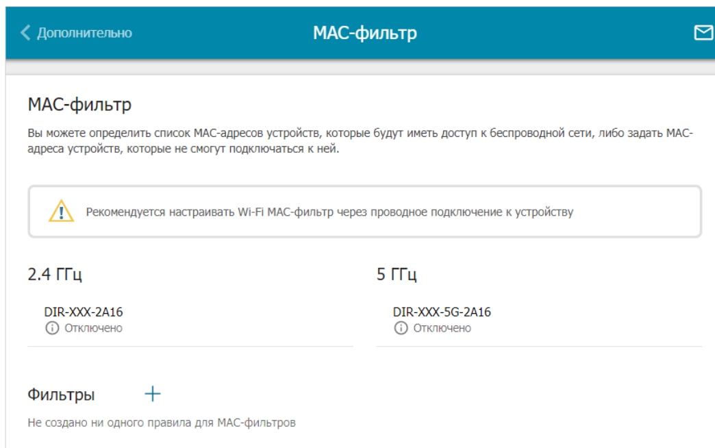
Рисунок 121. Страница для настройки MAC-фильтра для беспроводной сети.
