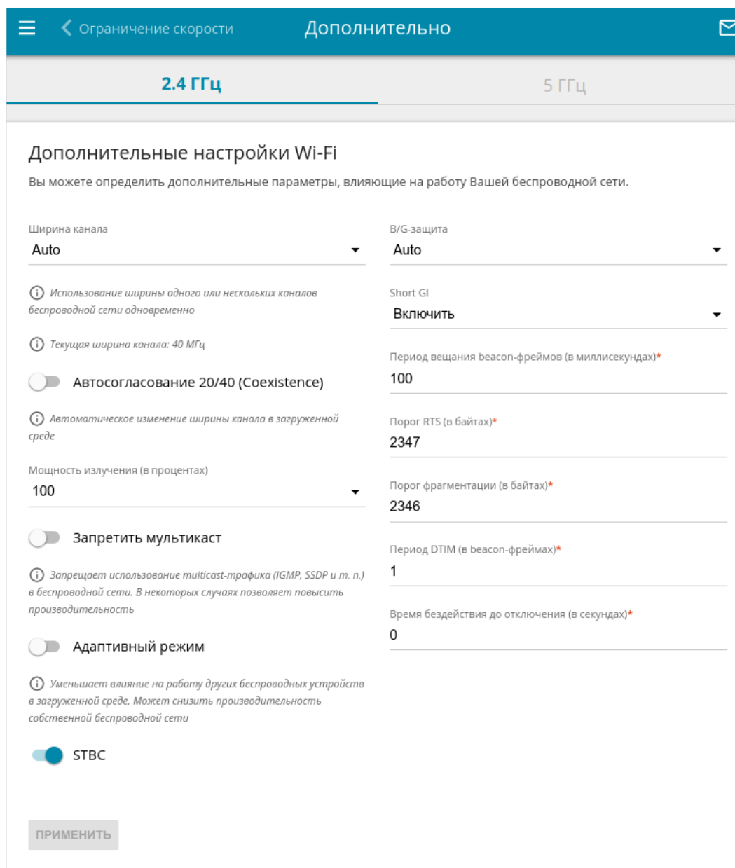
Рисунок 120. Страница дополнительных настроек для беспроводной сети.
