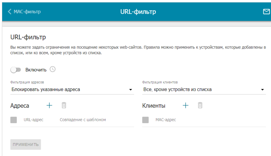
Рисунок 174. Страница Межсетевой экран / URL-фильтр .
