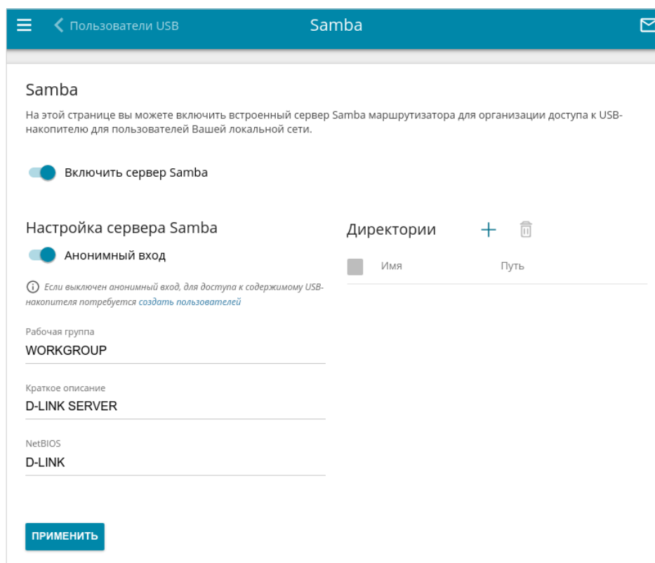
Рисунок 129. Страница USB-накопитель / Samba .
