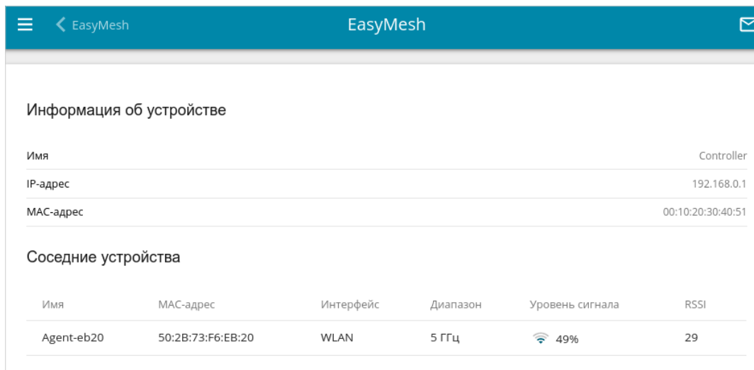
Рисунок 124. Страница с информацией об устройстве.
