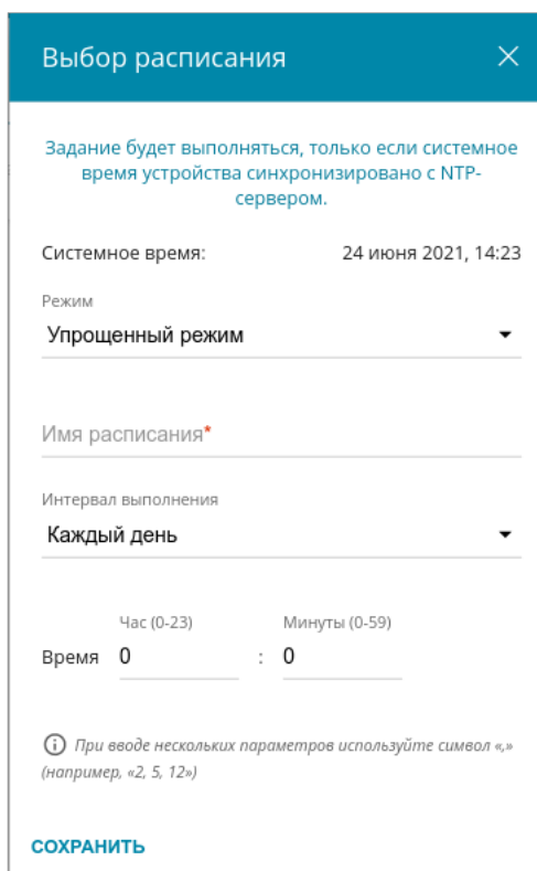
Рисунок 181. Окно настройки автоматической перезагрузки устройства по расписанию.
