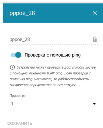
Рисунок 105. Окно изменения уровня приоритета соединения.
