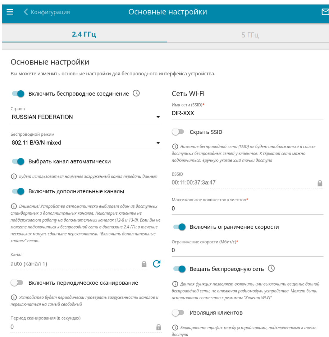
Рисунок 107. Основные настройки беспроводной локальной сети в диапазоне 2,4 ГГц.
