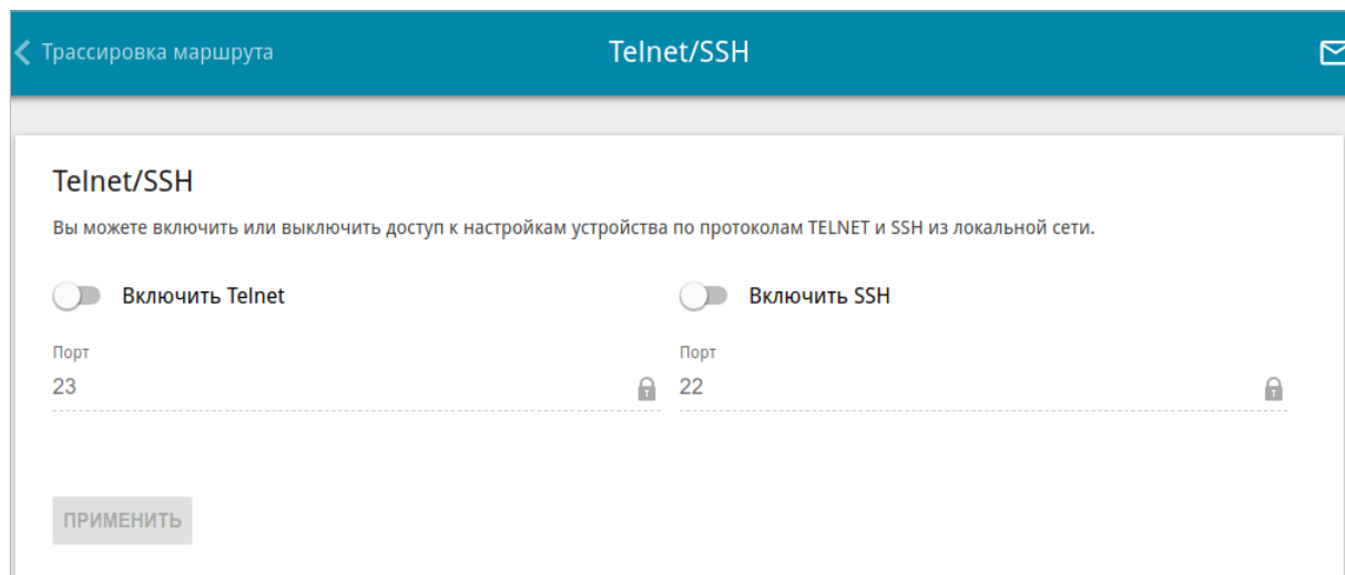
Рисунок 189. Страница Система / Telnet/SSH .
