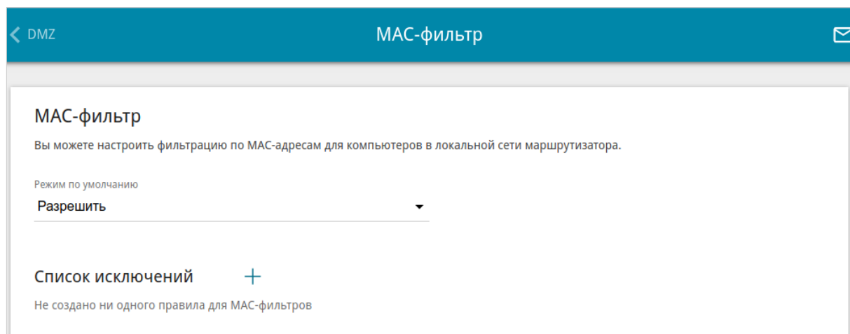
Рисунок 172. Страница Межсетевой экран / MAC-фильтр .
