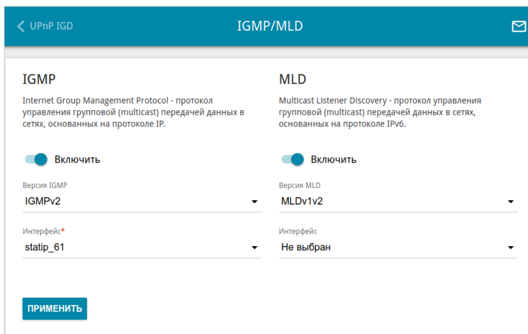
Рисунок 161. Страница Дополнительно / IGMP/MLD .
