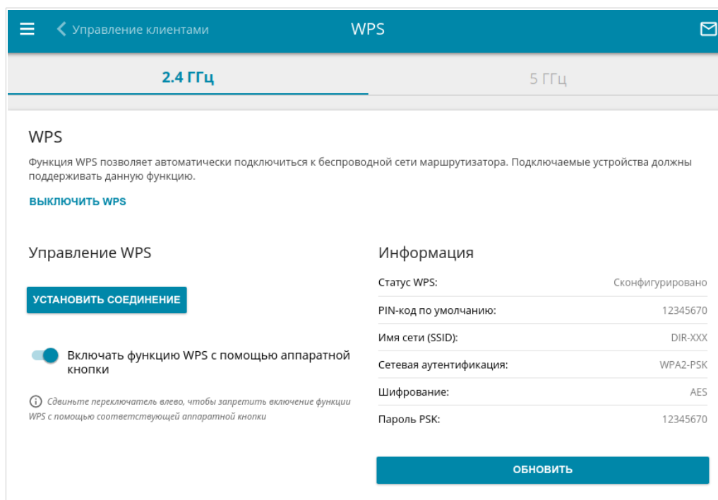
Рисунок 114. Страница для настройки функции WPS.
