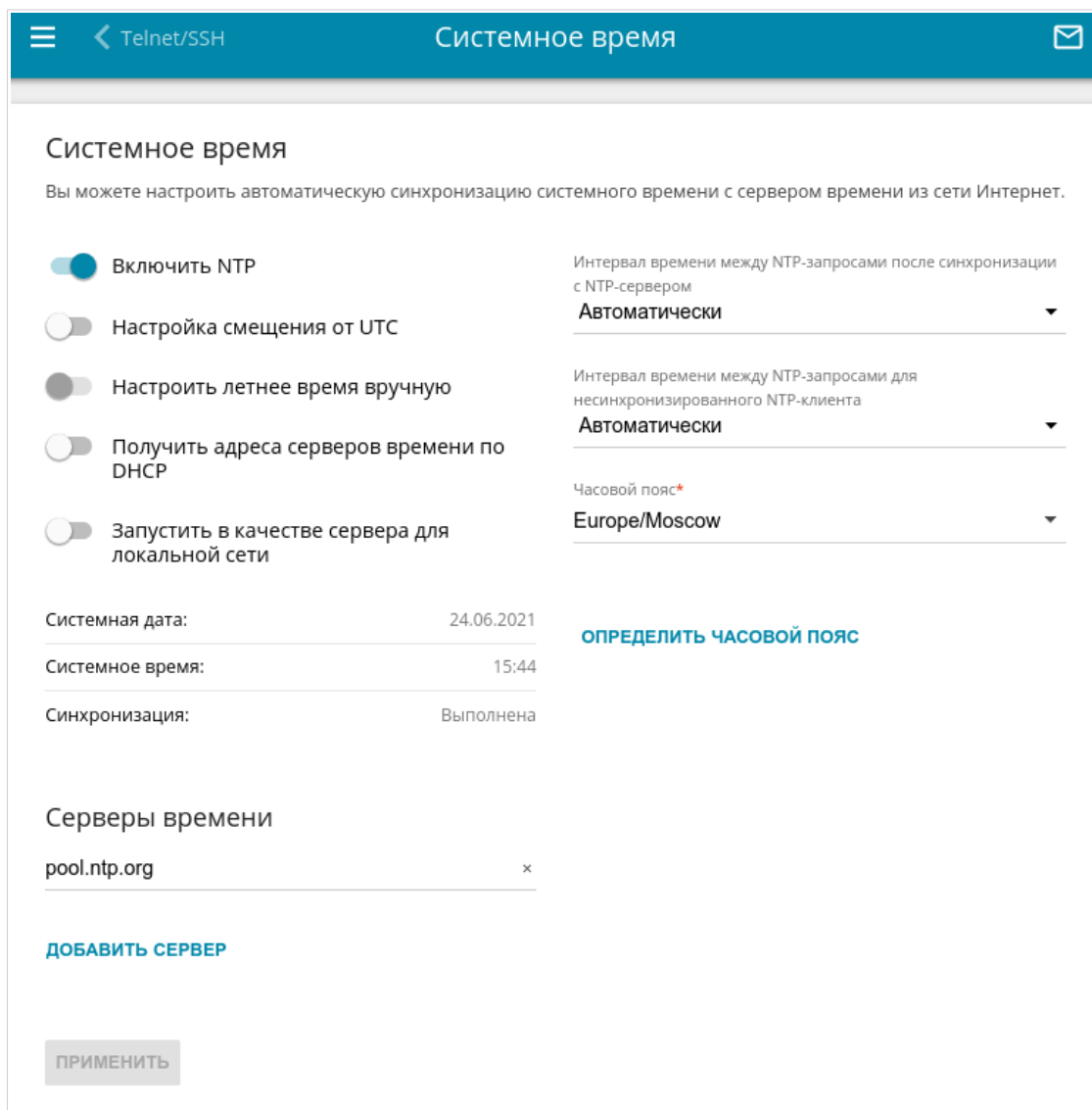
Рисунок 190. Страница Система / Системное время .
