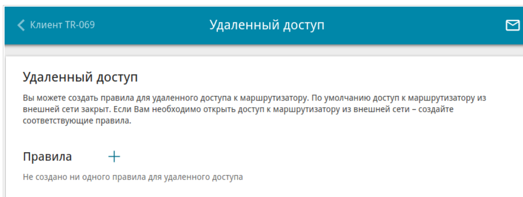
Рисунок 176. Страница Дополнительно / Удаленный доступ .
