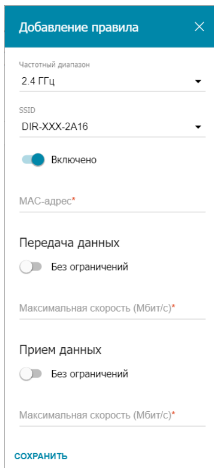
Рисунок 119. Окно для настройки ограничения скорости.
