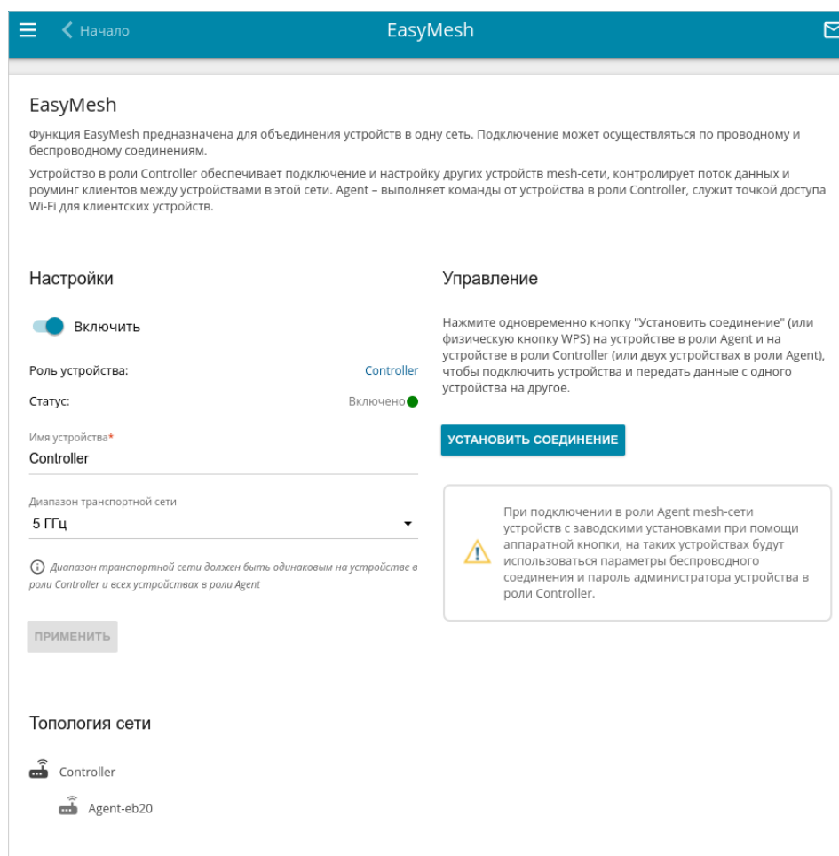
Рисунок 123. Страница Wi-Fi / EasyMesh .
