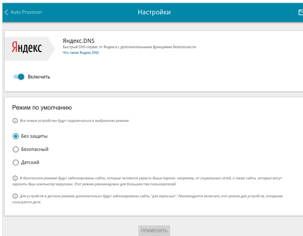
Рисунок 192. Страница Яндекс.DNS / Настройки .
