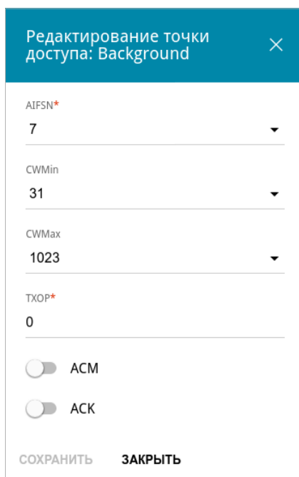
Рисунок 116. Окно для изменения параметров функции WMM.
