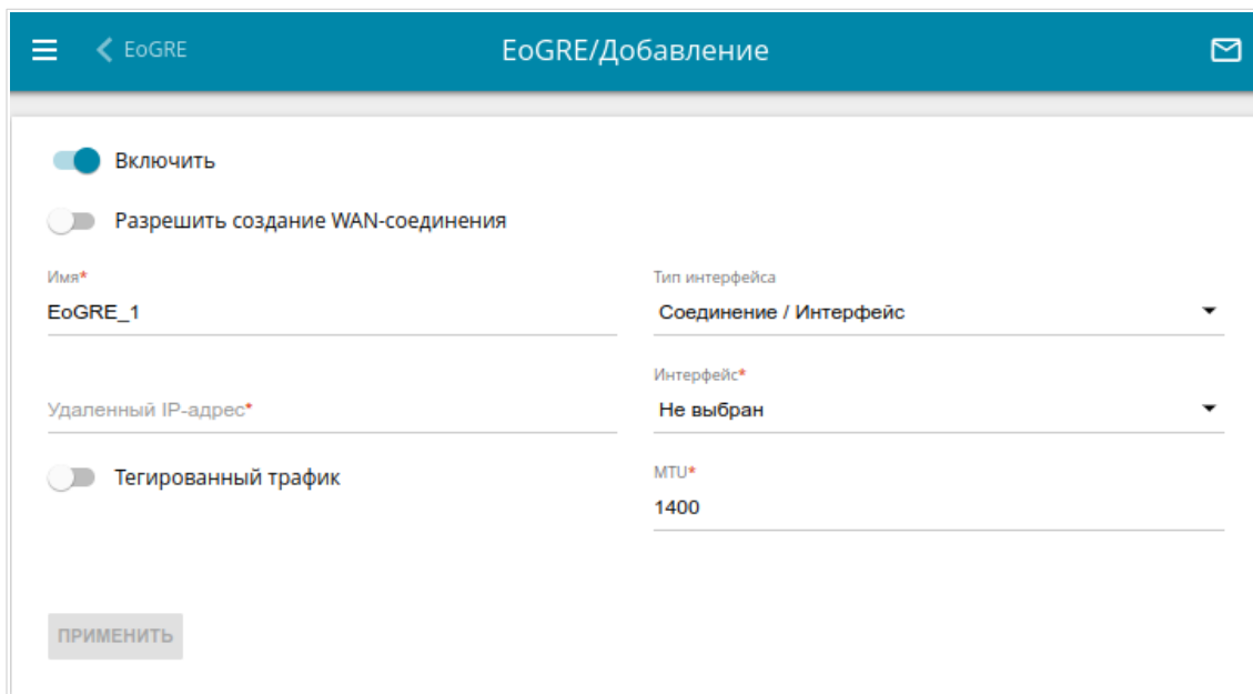
Рисунок 90. Страница добавления EoGRE-туннеля.
