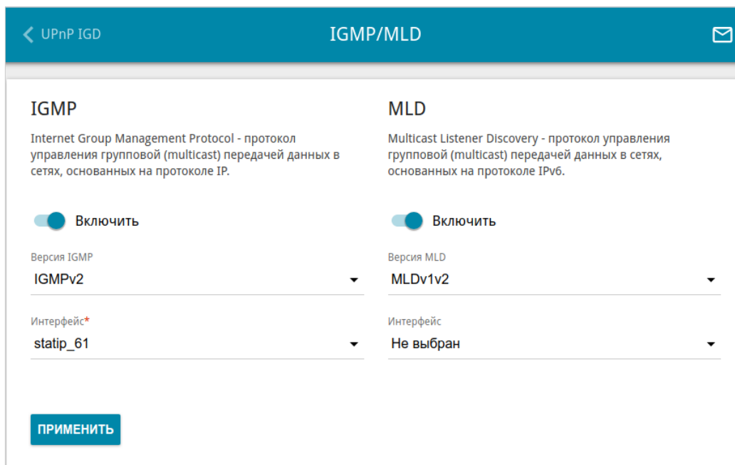
Рисунок 183. Страница Дополнительно / IGMP/MLD .
