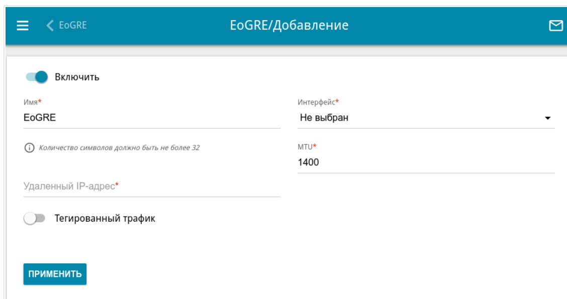
Рисунок 125. Страница добавления EoGRE-туннеля.
