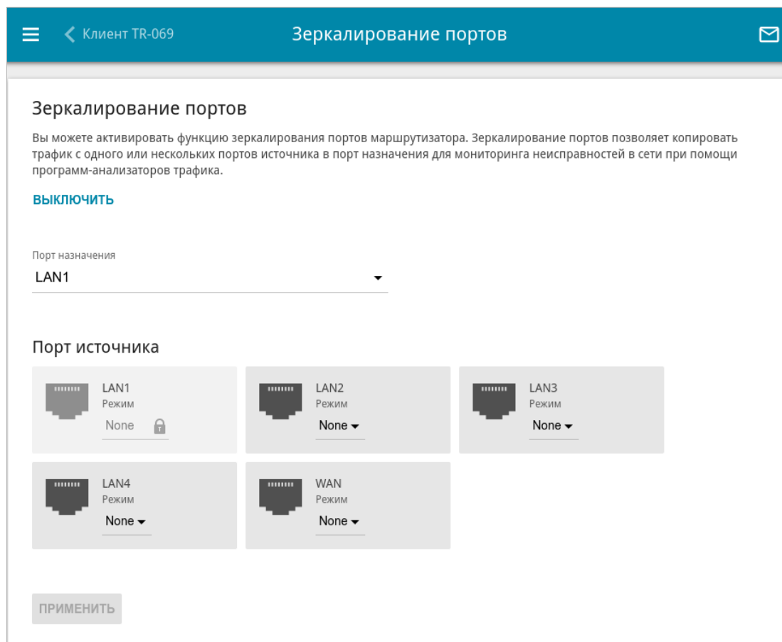
Рисунок 179. Страница Дополнительно / Зеркалирование портов .
