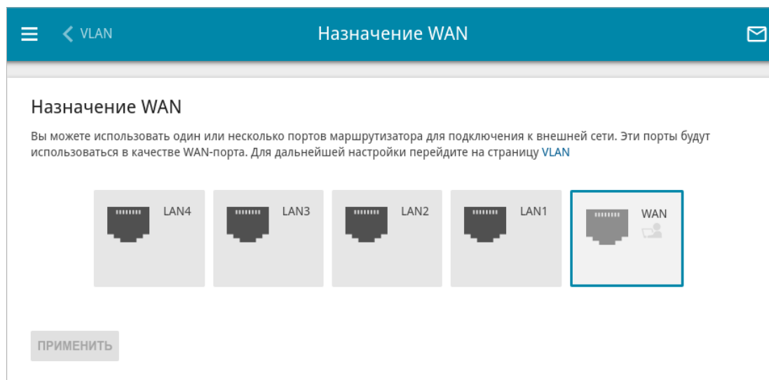
Рисунок 167. Страница Дополнительно / Назначение WAN .
